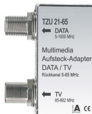
S 2165
